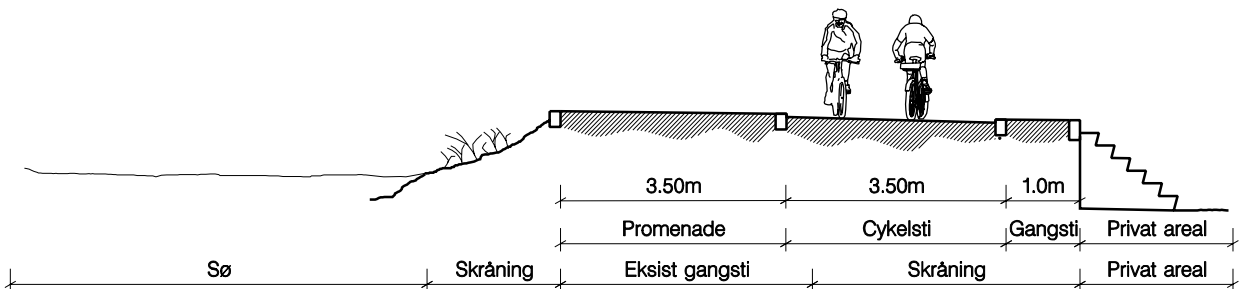
Principalsnit i strækning type C2
