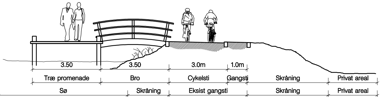
Principalsnit i strækning type C1
