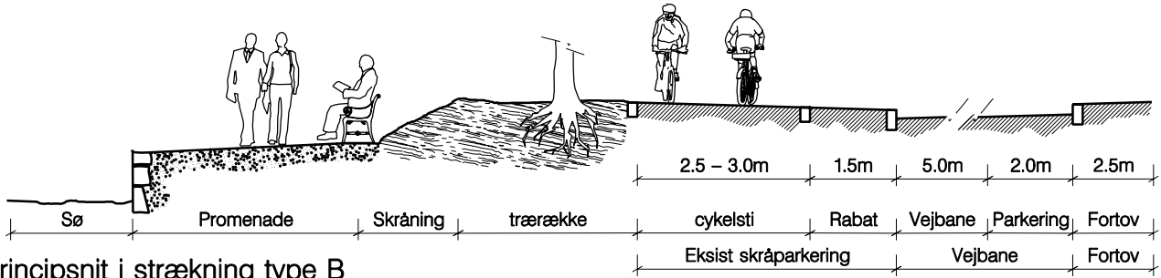
Principalsnit i strækning type B
